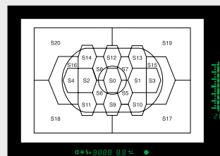
21zone 측광센서 분포도
