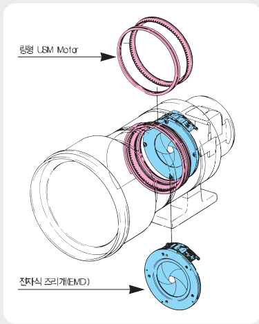
내장모터와 전자식 조리개
