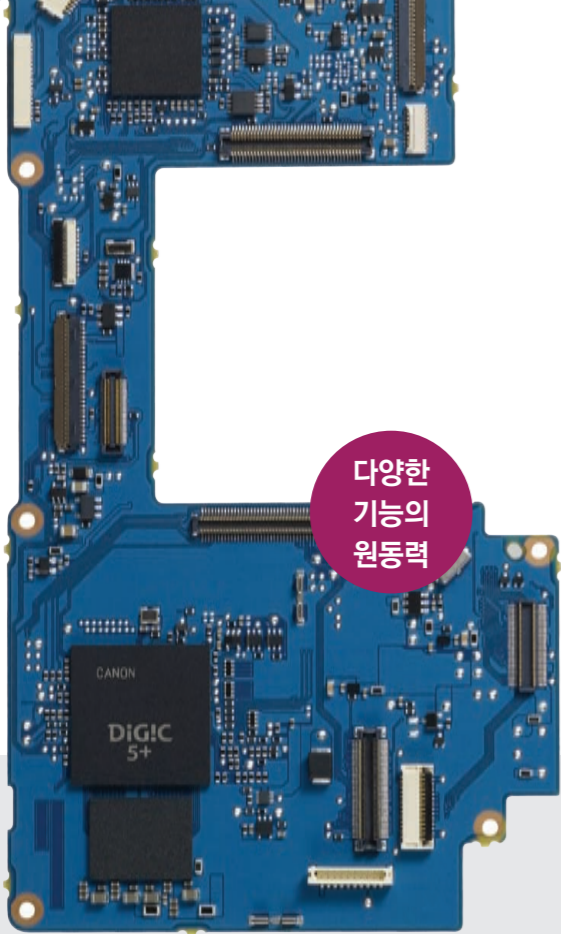
DIGIC 5+ 이미지 프로세서
